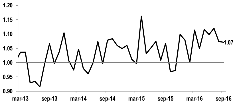
Cociente de nuevos pedidos sobre inventarios desestacionalizado
