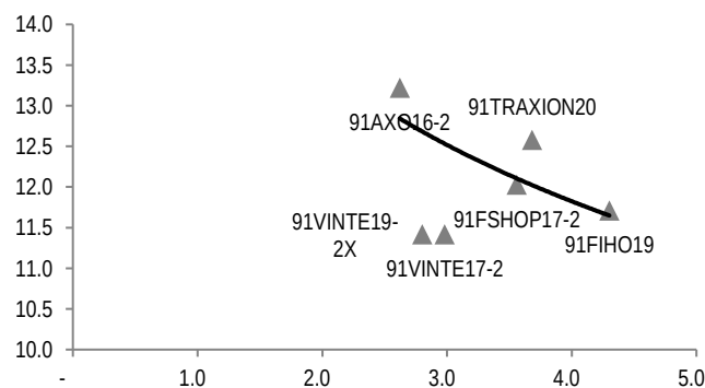
CIRCLEK 22-2 (Fija) – Relative Value Duración vs. YTM (%)
