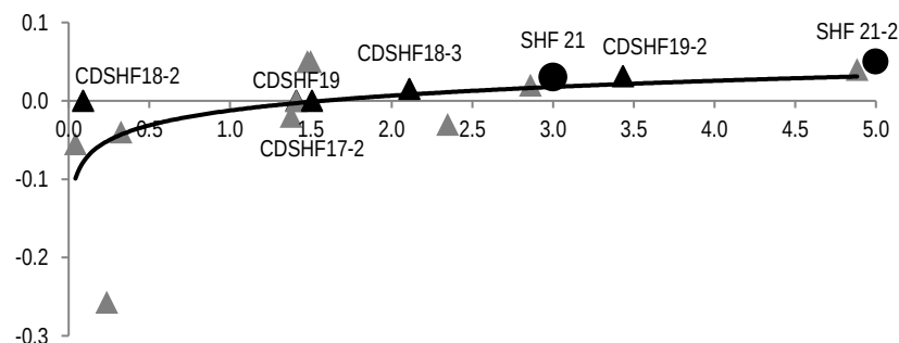
SHF 21 / 21-2 (TIIE 28) – Relative Value AxV vs. Sobretasa (%)
